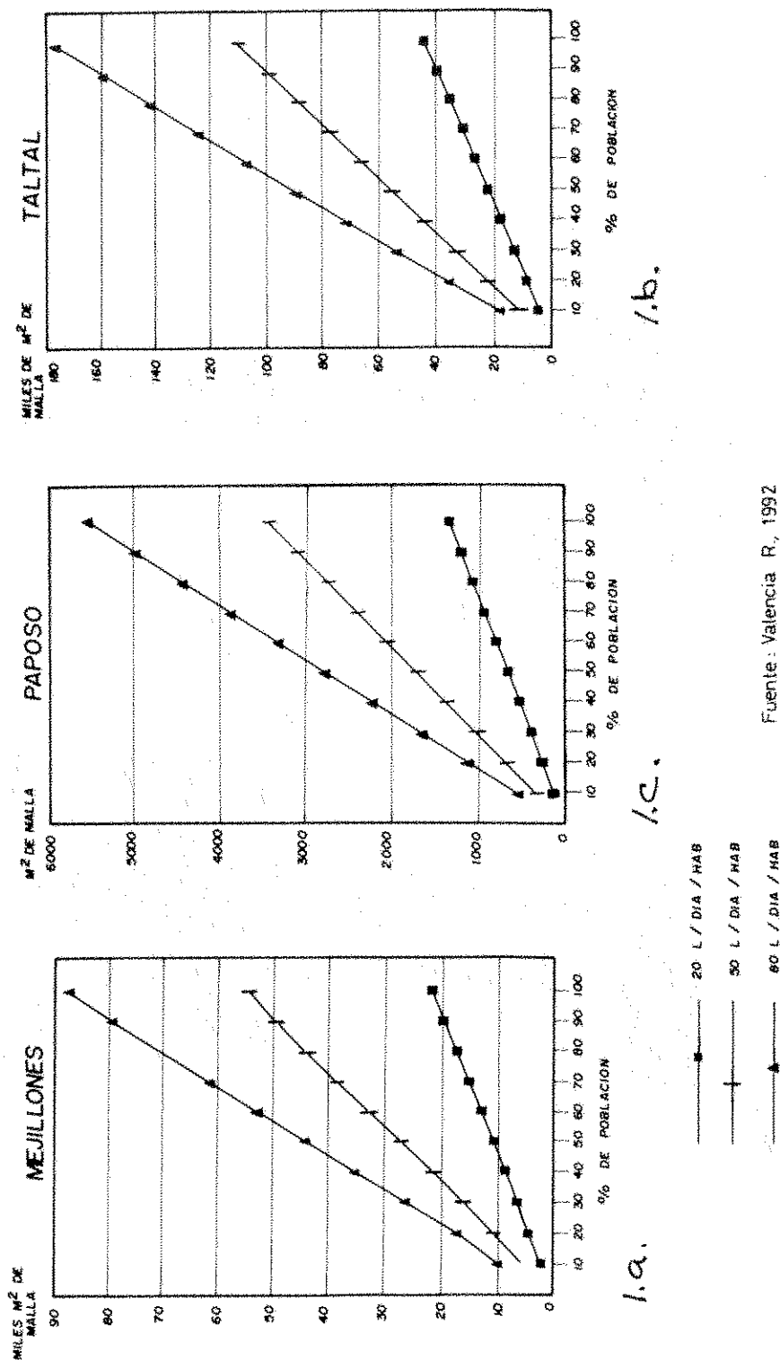
FIGURA N°1 ABASTECIMIENTO DE AGUA SEGUN DIFERENTES REQUERIMIENTOS Y LOCALIDAD MEJILLONES, PAPOSO Y TALTAL : 3.5 LIT / M2 / DIA
