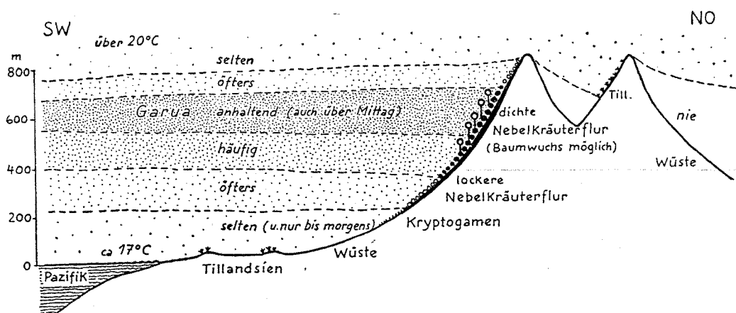
Abb. 1. Schematischer Schnitt durch eine peruanische Küstenloma. Häufigkeit des Hochnebels (garua) und Vegetationsverteilung im Südwinter.
