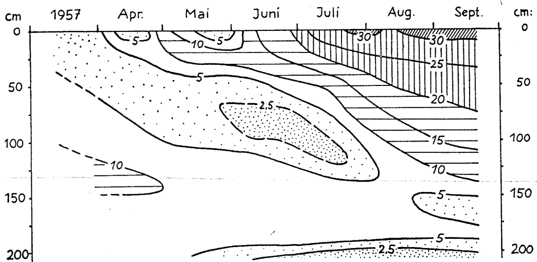
Abb. 7. Änderungen der Bodenfeuchtigkeit unter lockerem Eucalyptus -Bestand in den Lomas von Lachay. Im Jahre 1957 begann die nebelreiche Zeit ausnahmsweise erst im Juni.
